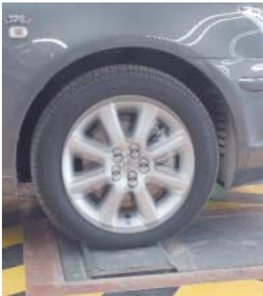
Equipo de placas oscilantes para la comprobación de la suspensión.
