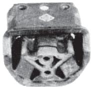
727 soporte motor dcho. 1.6D y 1.7D r.o.684267-684265
