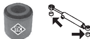
2911 silentbloc pistón cremallera asistida hasta '96, r.o. 4059.10 (12x24x20x24)
