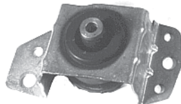
2343 soporte motor delantero derecho 1.4-1.6 r.o. 7610541
