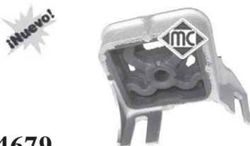
4679 soporte escape 1.5DCi r.o. 7700435270
