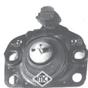
997 hidráulico: peso 1.430 g soporte motor derecho 1.4 desde '91 r.o. 7700805123
