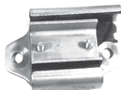
2467 soporte cambio VANETTE (hasta '93) y TRADE2.0,r.o.11320-Y9501
