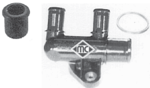
3523 racor conexión manguitos 1.6-1.8-2.0 r.o. 1336.J7-1336.H7
