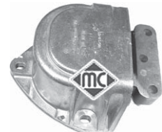
4790 soporte motor derecho 1.4TDi r.o. 6N0199867BF
