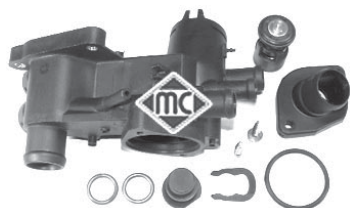
3615 cuerpo de termostato 1.0-1.4-1.6 completo con termostato ,r.o.032121111N
