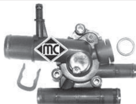
3569 CON TERMOSTATO cuerpo de termost. completo con accesorios 1.9D-DTi hasta '99, r.o. 7701474249
