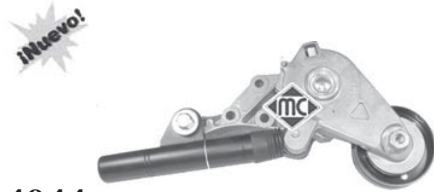
4944 tensor correa alternador 1.9TDi r.o.038903315C
