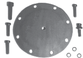
832 jgo reparación membrana depresor Diesel r.o.068198821A
