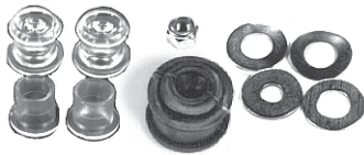
907 juego casquillos levas cambio TXE-DIESEL r.o. 7700689713+7700692252
