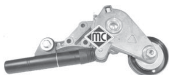
4944 tensor correa alternador 1.9TDi desde '97- r.o.038903315C
