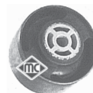
2869 silentbloc soporte posterior motor 1.6-1.8- 2.0, r.o. 1809.16
