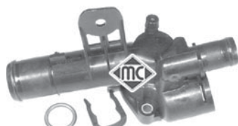
3679 caja con termostato 1.5DCi desde 7/03 r.o. 8200267349
