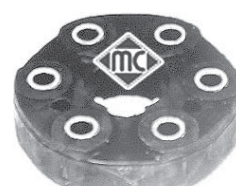
4347 Ø ext. 143 mm- Ø montaje 105 mm flector transmisión serie 3 E36, serie 5 E34 y E39 y serie 7, r.o. 26111229065
