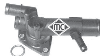
3670 caja con termostato 1.5DCi hasta 7/'03 r.o. 8200374994
