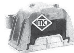
4368 soporte motor derecho 1.4-1.6 (de 105cv) -1.6/16v y 2.3V5, r.o. 1J0199262BK/BH
