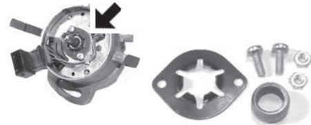
4296 kit reparación distribuidor Magneti-Marelli (casquillo sinterizado del eje rotor)
