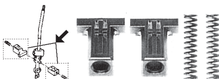
2303 juego casquillos palanca cambio (5 veloci- dades desde '87), r.o. 6172154
