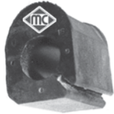
868 para barra de Ø 23 mm goma central barra estabilizadora r.o. 7700785788
