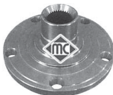
90054 38 estrías bujes rueda delantera 1.9TDi (AFN) y 2.8 r.o. 4A0407615D
