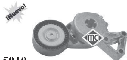
5010 tensor correa alternador 1.8 desde '00- r.o. 06A903315E
