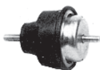
697/1 NO HIDRÁULICO (460 g.) soporte de motor derecho 1.1 - 1.4 y 1.8 r.o. ----
