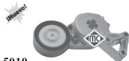
5010 tensor correa alternador 1.8 desde '00- r.o. 06A903315E
