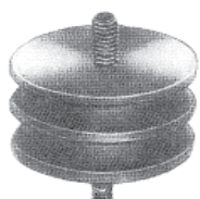
404 soporte de motor Ø 63 mm (rosca M-10) LANDROVER, r.o. 277513
