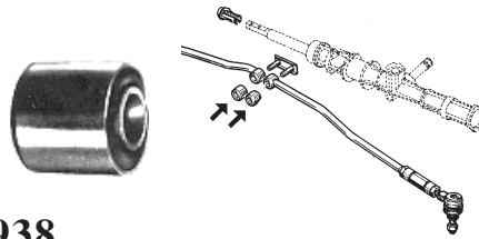
938 silentbloc barras dirección TXE-DIESEL r.o. no hay despiece (10x23x19x24.5)
