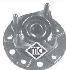
90005 bujes rueda delata 1.8-2.0 hasta '95 y 1.7D-TD de 33 estrías, Ø disco 66 mm, r.o. 326184
