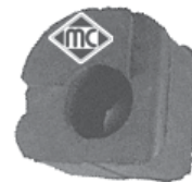
4266 goma para barra estabilizadora de Ø 20 mm r.o. 1H0411314
