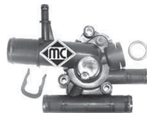
3645 caja de termostato completa desde '99 (89°) r.o. 8200074346
