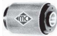
2801 (16x50.5x82x61) silentbloc posterior inferior ballesta trasera r.o. 6191746
