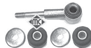
2948 bieleta puntal barra estabilizadora completa Expert y 806, r.o.5087.35
