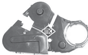
3698 juego tapas correa distribución 1.9 XUD r.o. 0320.H2+0320.H3+0320.F9
