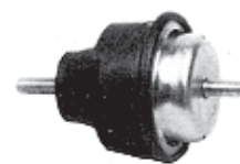
697/1 no hidráulico (460 g.) soporte de motor derecho 1.4 y 1.8 r.o. ----
