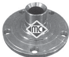
90053 33 estrías bujes rueda delantera todos modelos salvo 1.9TDi (motor AFN) y 2.8, r.o. 8D0407615E
