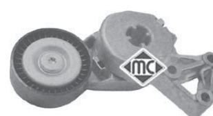
5010 tensor correa alternador 1.6-1.8-2.0 r.o. 06A903315E
