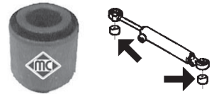
2911 silentbloc pistón cremallera asistida r.o.4059.10 (12x24x20x24)
