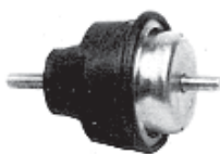
697 HIDRAULICO (650 g.) soporte de motor derecho 1.4 y 1.8 r.o. 1844.38
