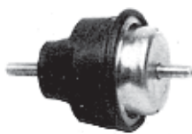
697 HIDRAULICO (650 g.) soporte de motor derecho 1.4-1.6 r.o. 1844.38
