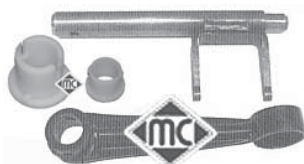
4300 horquilla embrague completa con casquillos motores TU, r.o. 2117.52
