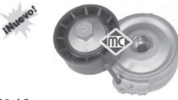
5043 rodillo de Ø 60 mm tensor correa alternador 2.0 HDi r.o. 5751.74
