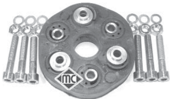
953 flector de transmisión (Øext. 127 mm), r.o. 1244100015
