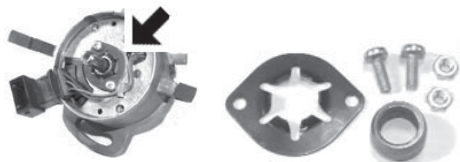
4296 kit reparación distribuidor Magneti-Marelli (casquillo sinterizado del eje rotor)
