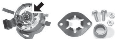
4296 kit reparación distribuidor Magneti-Marelli 1.4-1.6 (casquillo sinterizado del eje rotor)
